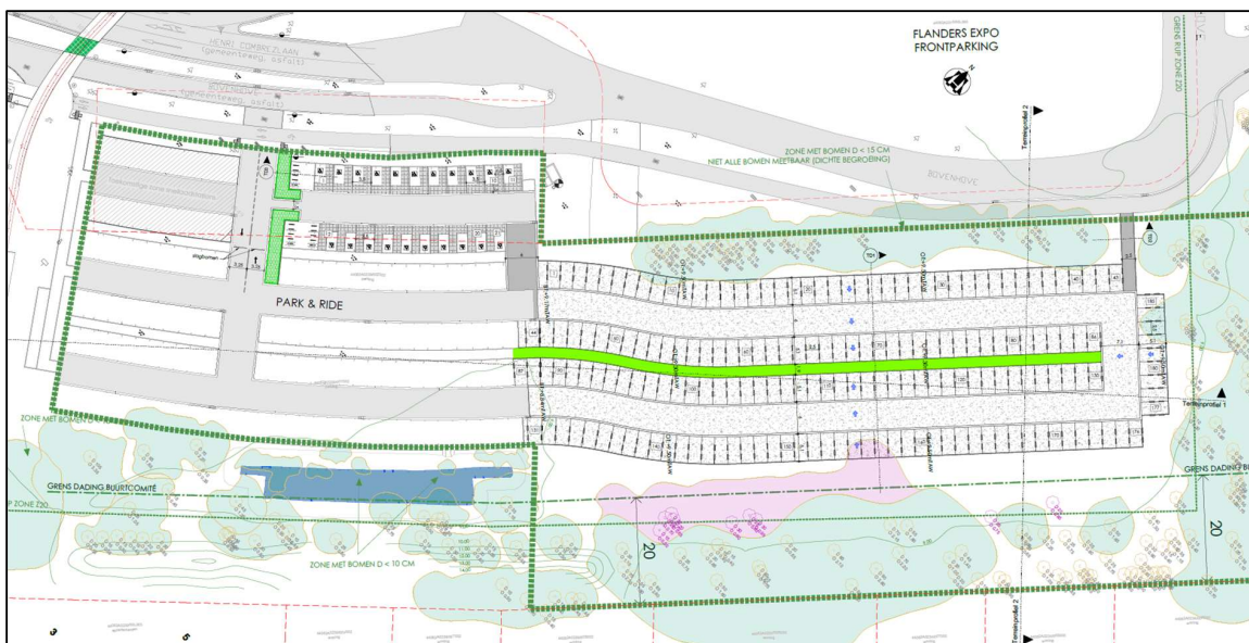
Figuur 4 - Ontwerpplan maaiveldparking (bestaand + uitbreiding)
