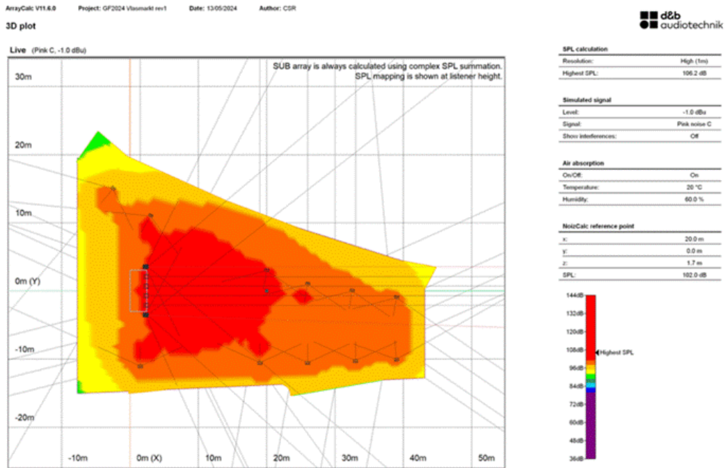
De NoizCalc simulatie in dB(C)
