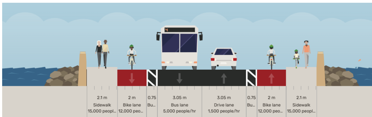
Figuur 8: Scenario 1c, TDP volgens randvoorwaarden
