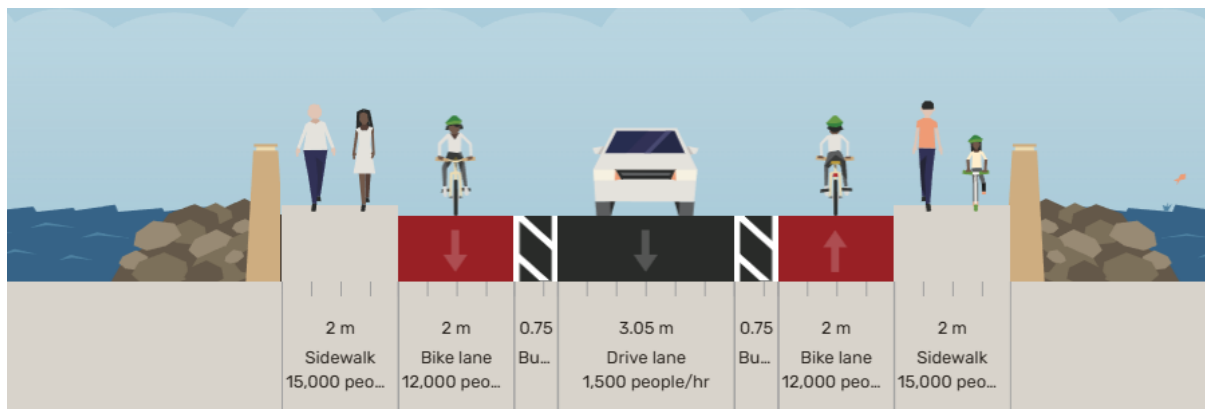
Figuur 8-23: Scenario 3a, TDP standaardbrug 12,6m
