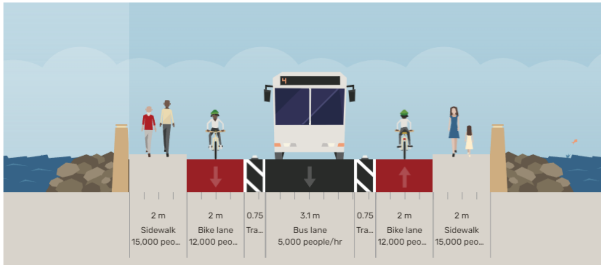
Figuur 11: Scenario 1d, TDP met een brug van 12,6m
