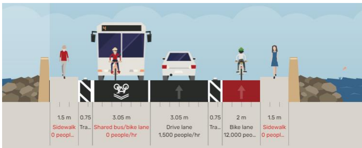
Figuur 13: Scenario 2a, TDP Wondelgemstraatbrug
