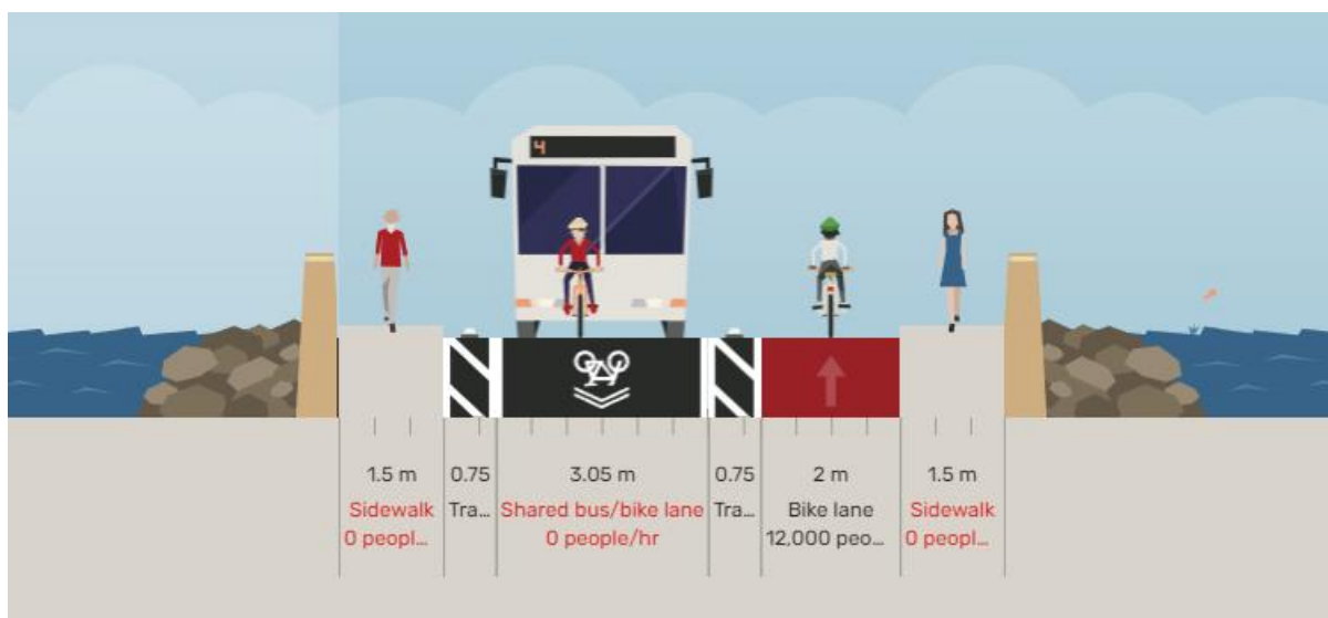
Figuur 8-10: Scenario 1d, TDP met een brug van 9,55m
