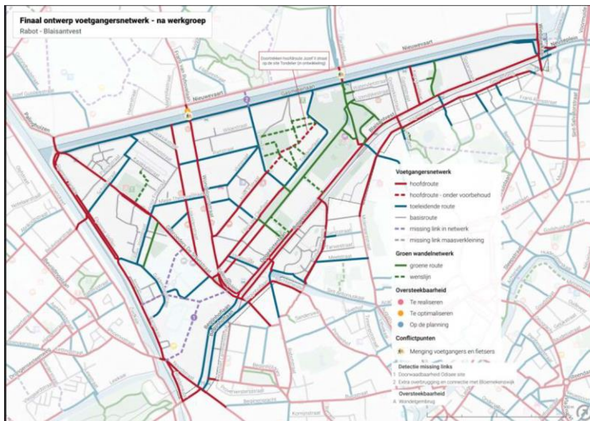
Figuur 2-8 Ontwerp van voetgangersnetwerk Rabot-Blaisantvest
