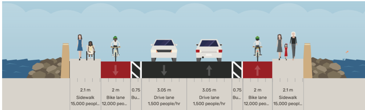
Figuur 3: Scenario 1a, TDP volgens randvoorwaarden
