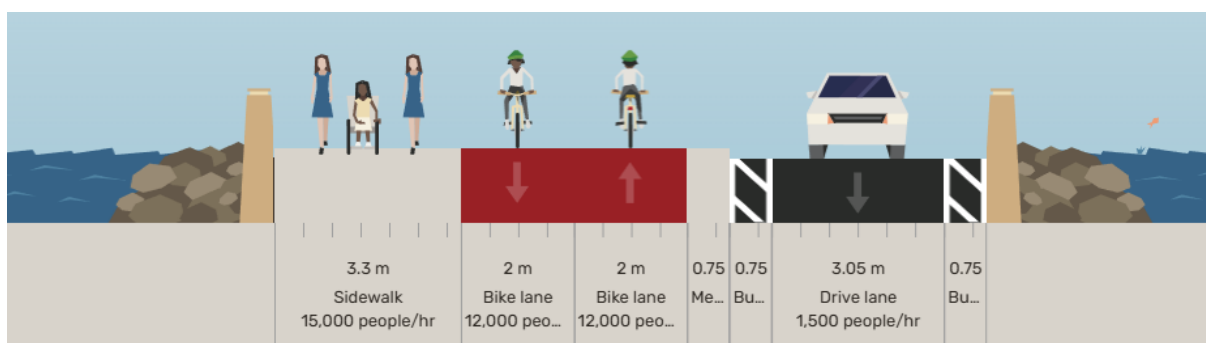
Figuur 14: Scenario 2a, TDP Nieuwe brug (westwaarts)
