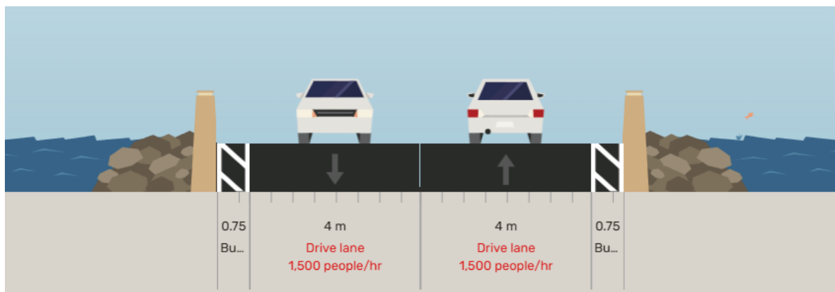
Figuur 8-20: Scenario 2c, TDP Wondelgemstraatbrug
