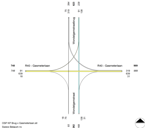
Figuur 4-10: Intensiteiten (pae) kruispunt Wondelgemstraatbrug x R40 Gasmeterlaan
