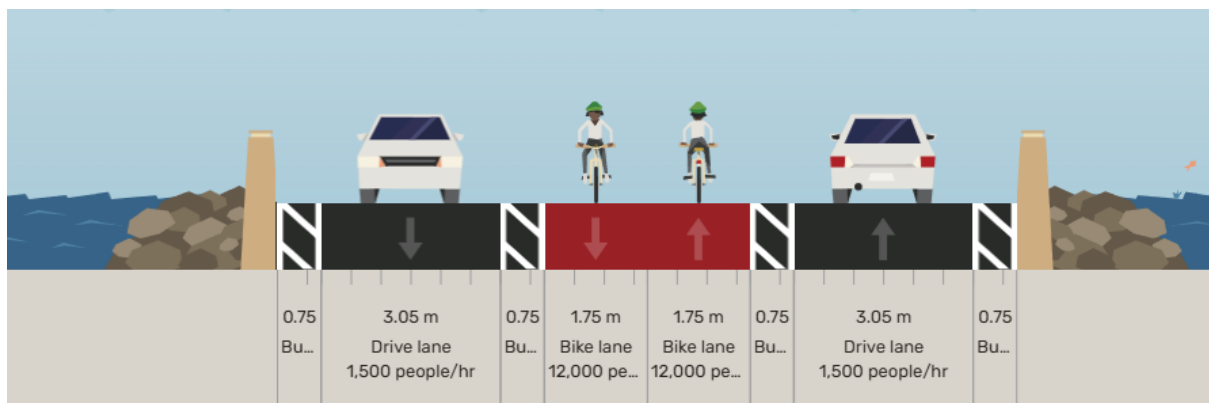
Figuur 17: Scenario 2b, TDP Nieuwe brug (westwaarts), rekening houdend met standaardmaten
