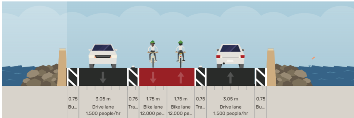
Figuur 28: Scenario 3b, TDP Nieuwe brug (westwaarts), rekening houdend met standaardmaten
