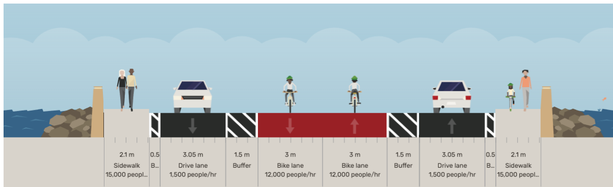
Figuur 8-18: Scenario 2b, TDP Nieuwe brug (westwaarts), rekening houdend met infrastructurele randvoorwaarden
