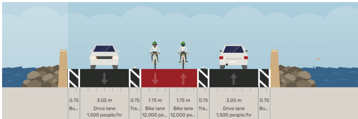
Figuur 24: Scenario 3a, TDP Nieuwe brug (oostwaarts), rekening houdend met standaardmaten
