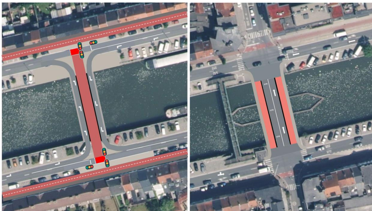
Figuur 8-15: concept oplossingsvoorstel 2b: Wondelgemstraatbrug: stad uit, Nieuw brug: U-turn in beide richtingen
