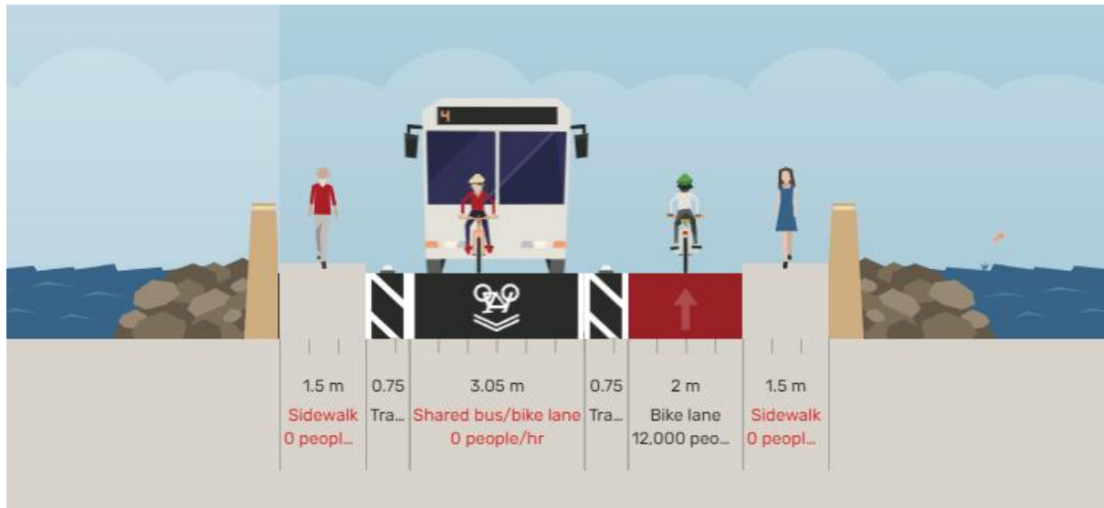
Figuur 8-27: Scenario 3b, TDP met een brug van 9,55m
