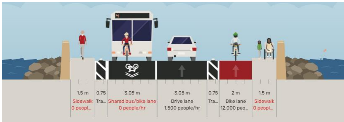
Figuur 16: Scenario 2b, TDP Wondelgemstraatbrug
