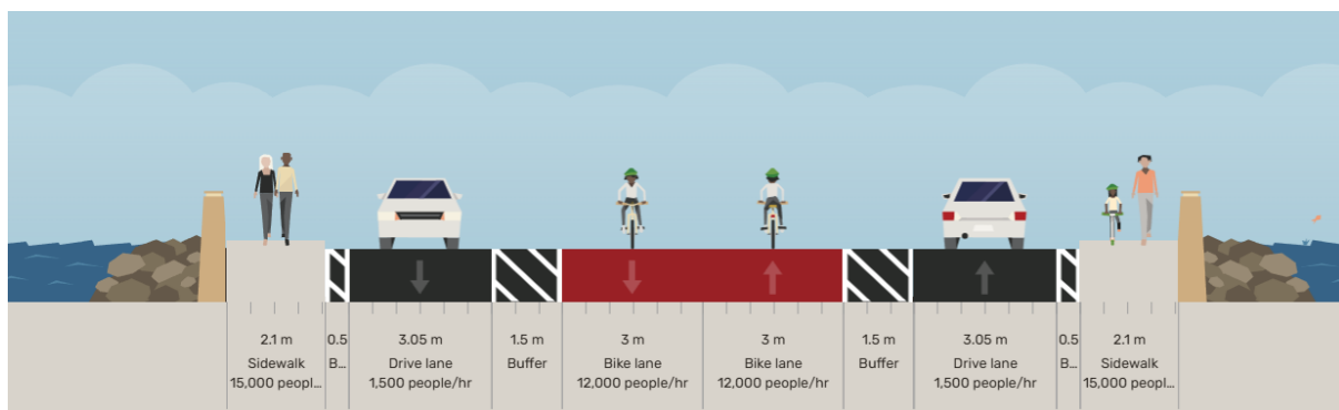
Figuur 8-29: Scenario 3b, TDP Nieuwe brug (westwaarts), rekening houdend met infrastructurele randvoorwaarden
