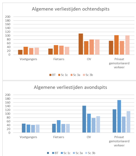
Figuur 31: Algemene verliestijden scenario's
