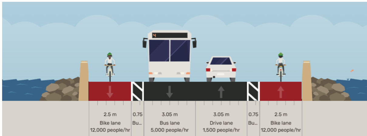
Figuur 7: Scenario 1c, TDP standaardbrug 12,6m
