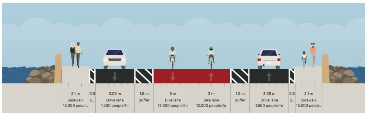
Figuur 8-25: Scenario 3a, TDP Nieuwe brug (oostwaarts), rekening houdend met infrastructurele randvoorwaarden
