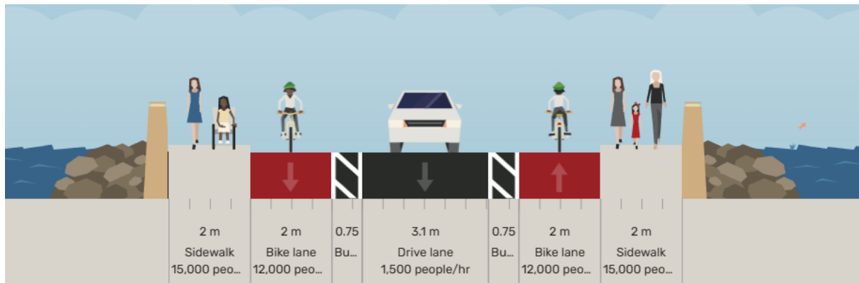
Figuur 8-5: Scenario 1a, TDP standaardbrug 12,6m
