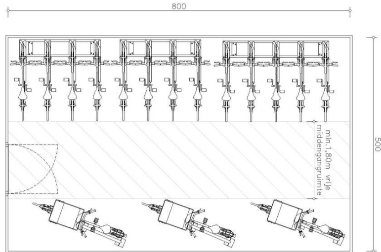
Figur 3: Voorbeeld van een basismodule voor: 13 standaard fietsen + 3 fietsen met afwijkende afmetingen
