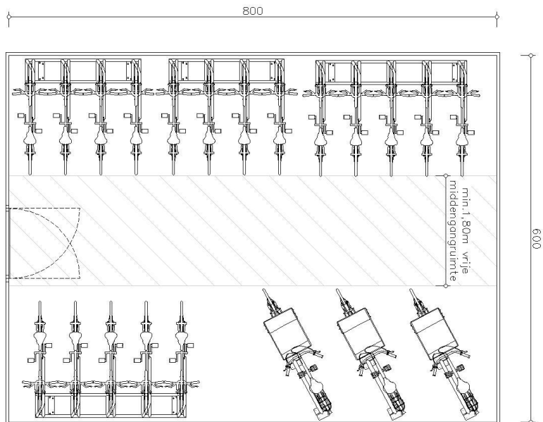
Figur 4: Voorbeeld van een basismodule voor: 18 standaard fietsen + 3 fietsen met afwijkende afmetingen
