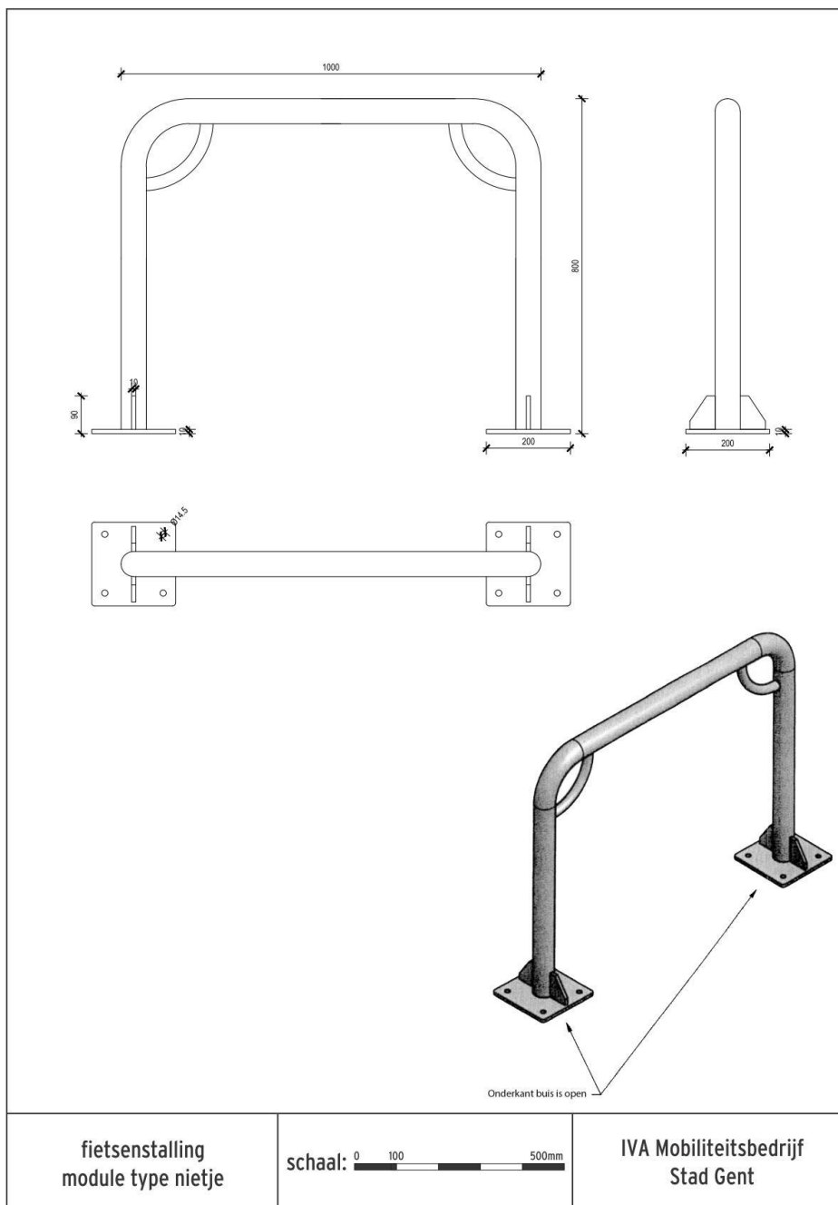
Figuur 6: Module Type Gent Nietje – technische tekening.
