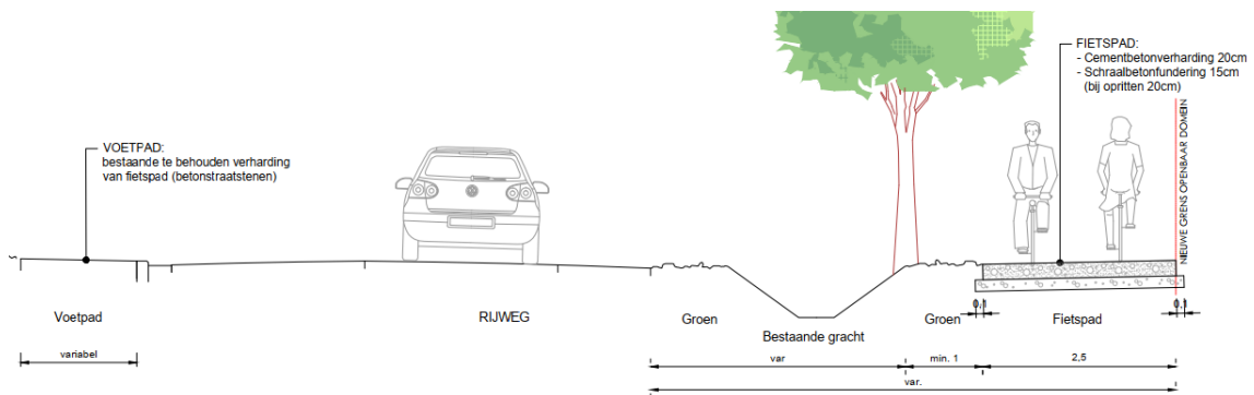
TYPEDWARSPROFIEL 7 - Schaal 1/50
