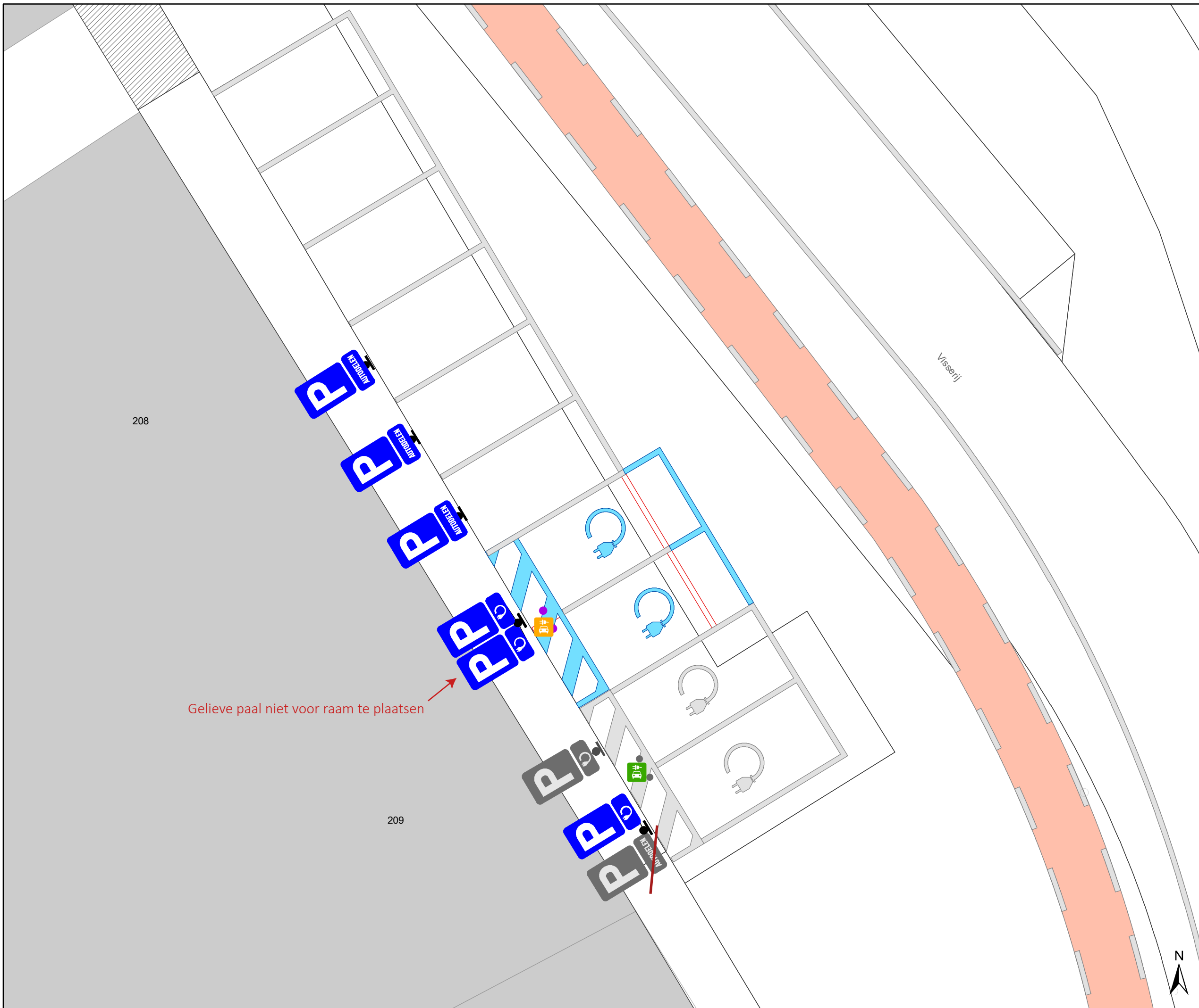
Geplande signalisatie
